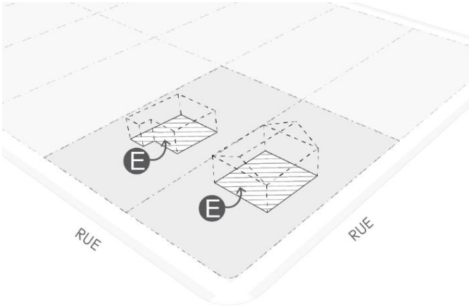
Figure 1 Mesure de la superficie d’implantation d’un bâtiment
