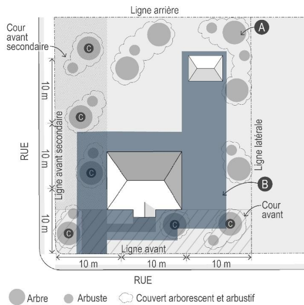
Figure 236 Aménagement d'un terrain
