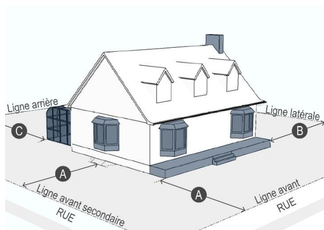
Figure 200 Éléments architecturaux d'un bâtiment principal
