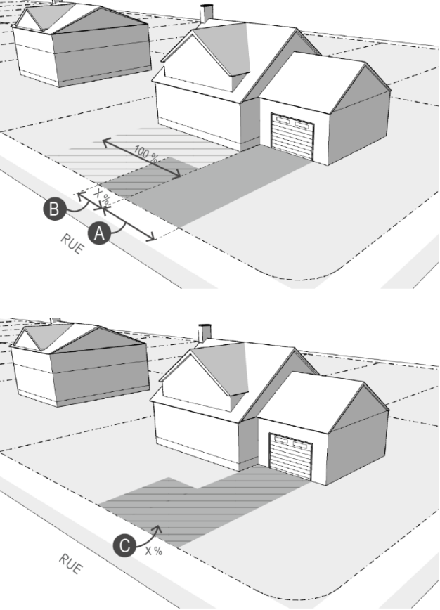
Figure 237 Aménagement d'une aire de stationnement
