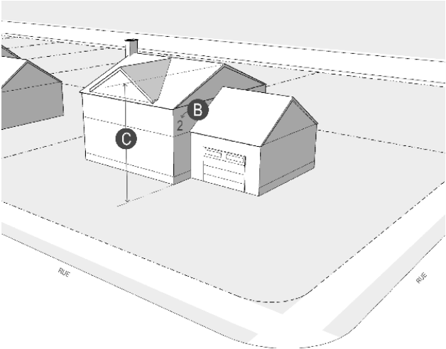
Figure 156 Hauteur d'un bâtiment
