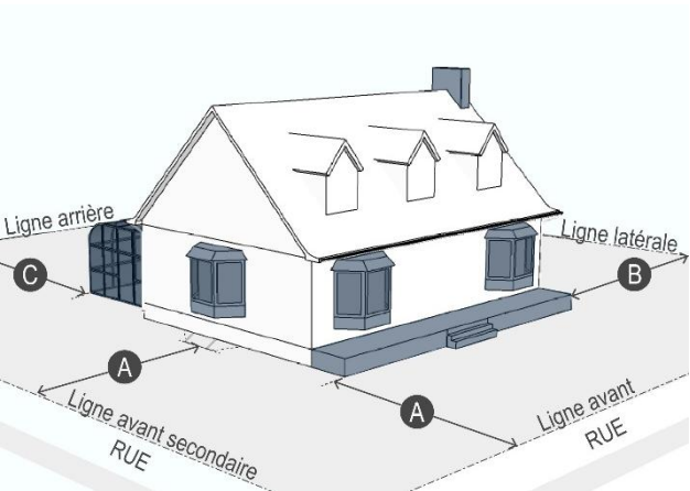
Figure 149 Éléments architecturaux d'un bâtiment principal
