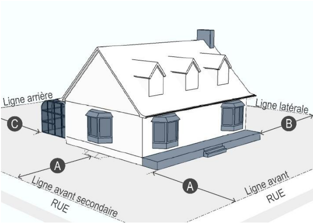
Figure 168 Éléments architecturaux d'un bâtiment principal
