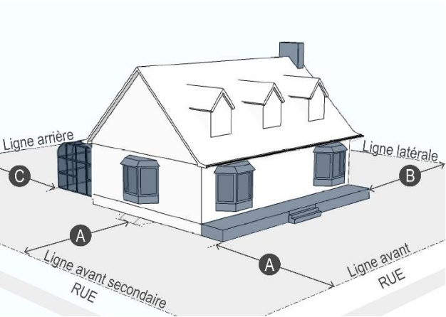
Figure 133 Éléments architecturaux d'un bâtiment principal
