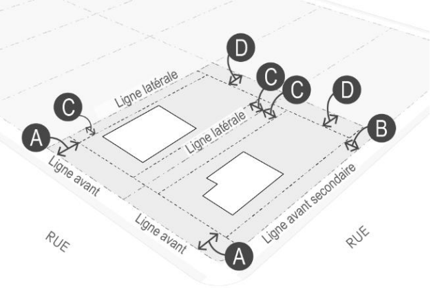
Figure 213 Marges de recul
