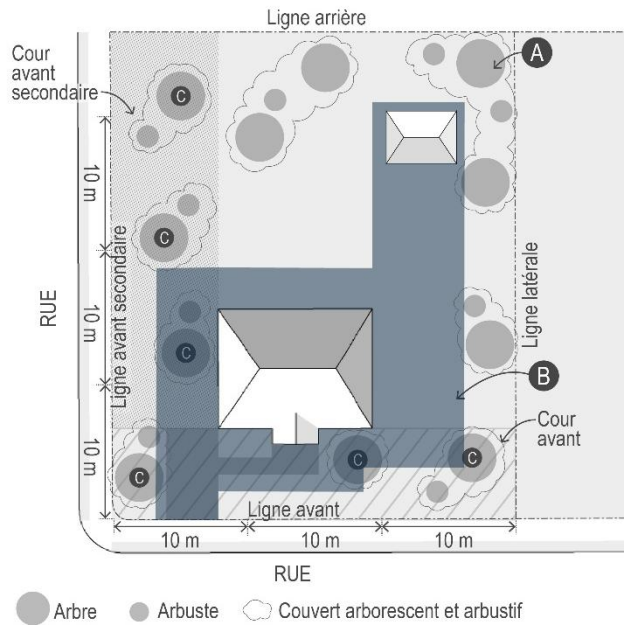
Figure 169 Aménagement d'un terrain
