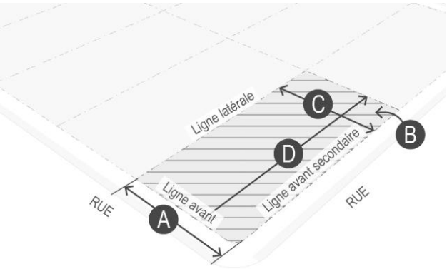
Figure 48 Normes de lotissement
