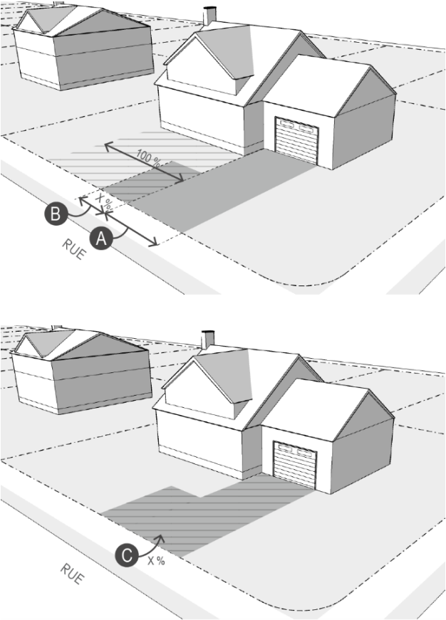
Figure 39 Aménagement d'une aire de stationnement
