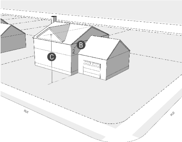
Figure 36 Hauteur d'un bâtiment
