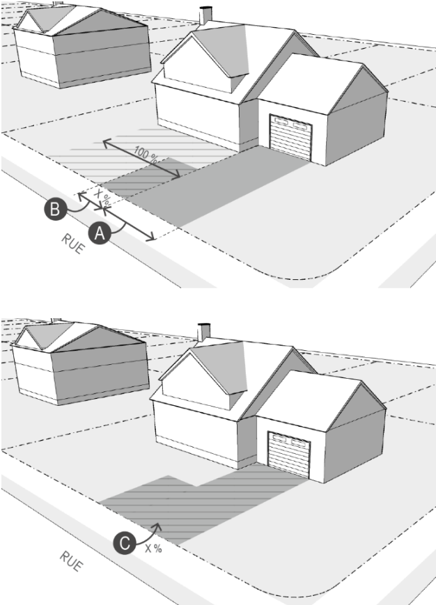
Figure 186 Aménagement d'une aire de stationnement
