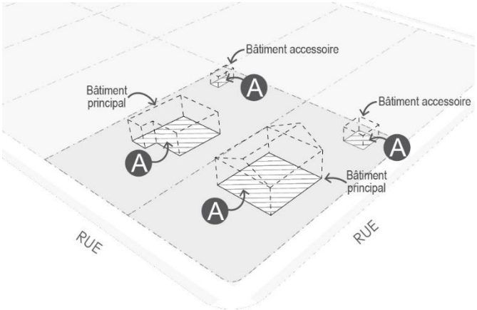
Figure 20 Mesure de l’emprise au sol de tous les bâtiments
