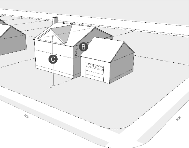
Figure 156 Hauteur d'un bâtiment
