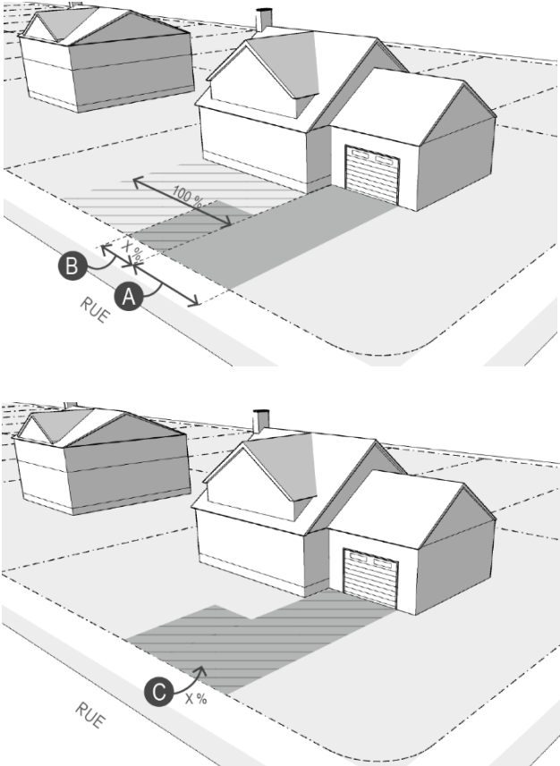
Figure 159 Aménagement d'une aire de stationnement
