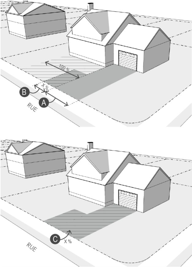
Figure 210 Aménagement d'une aire de stationnement
