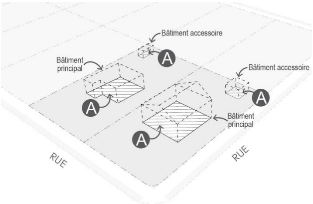
Figure 66 Emprise au sol totale du bâtiment principal et des bâtiments accessoires
