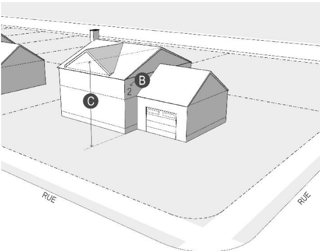
Figure 226 Hauteur d'un bâtiment
