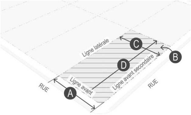
Figure 32 Normes de lotissement
