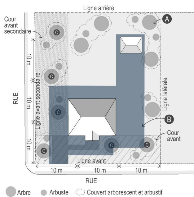
Figure 220 Aménagement d'un terrain
