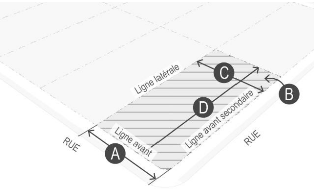
Figure 179 Normes de lotissement
