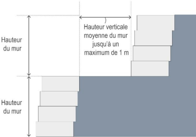
Figure 286 Coupe de mur de soutènement aménagé en palier
