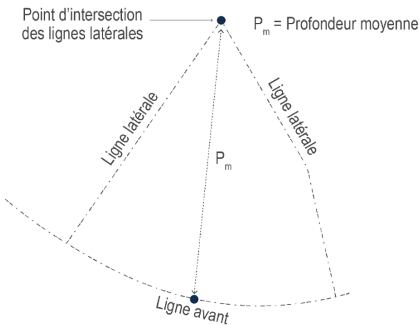
Figure 10 Calcul de la profondeur moyenne lorsqu'il n'y a pas de ligne arrière
