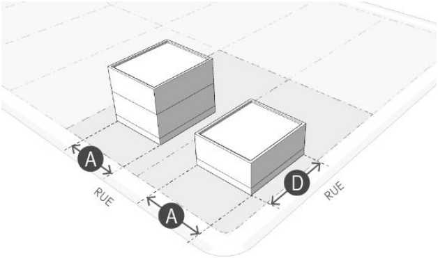
Figure 206 Largeur et profondeur d'un bâtiment
