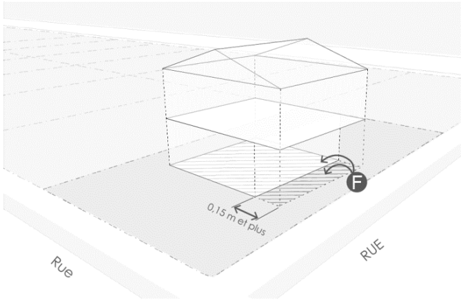
Figure 21 Mesure de l’emprise au sol d’un bâtiment en présence d’une saillie
