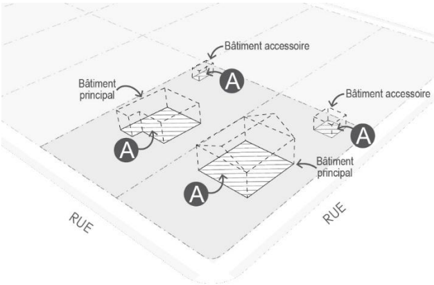
Figure 154 Emprise au sol totale du bâtiment principal et des bâtiments accessoires
