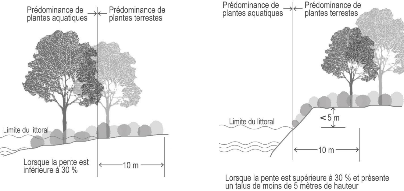
Figure 6 Mesure d'une rive d'une largeur de 10 m
