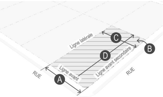
Figure 187 Normes de lotissement
