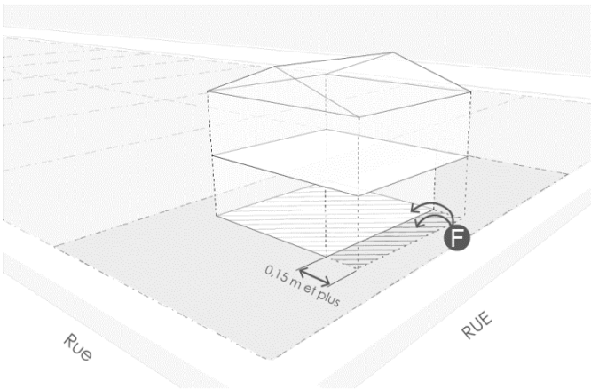
Figure 2 Mesure de l'emprise au sol du bâtiment en présence d'une saillie
