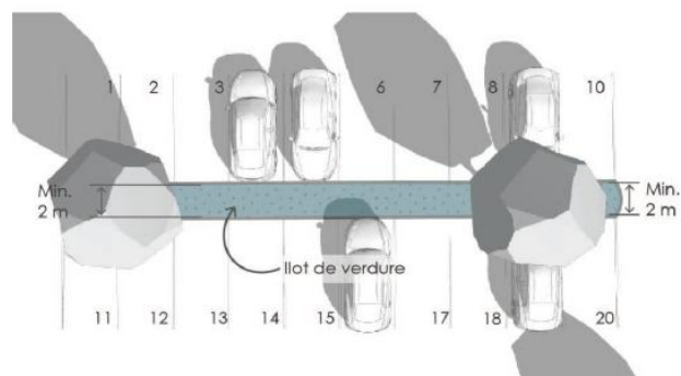
Figure 283 Aménagement des îlots de verdure – Proposition « A »
