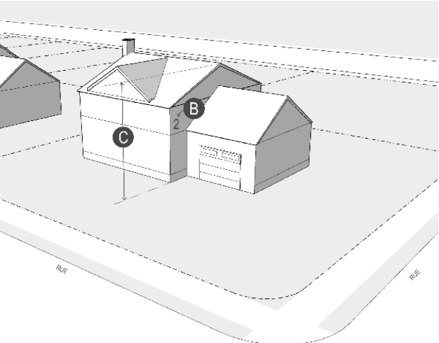
Figure 92 Hauteur d'un bâtiment
