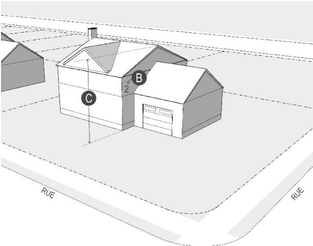
Figure 218 Hauteur d'un bâtiment
