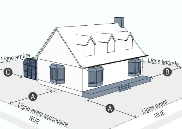
Figure 109 Éléments architecturaux d'un bâtiment principal
