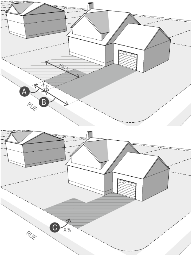
Figure 178 Aménagement d'une aire de stationnement
