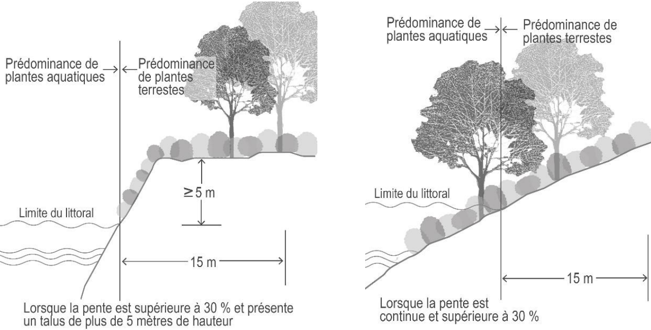
Figure 7 Mesure d'une rive d'une largeur de 15 m
